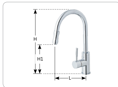
A-2066A $10,000 單槍抽取式廚房混合龍頭（檯面上） 尺寸(mm): H=370 H1=205 L=205 ※可抽取長度約450mm 適用水壓範圍0.5~5kgf/cm 2
