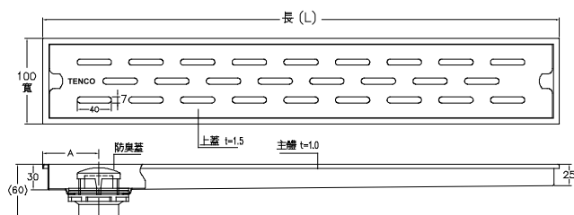
A-3703 300×100mm $5,400 A-3706 600×100mm $7,500 A-3708 800×100mm $9,800 A-3709 900×100mm $11,000 A-3710 1000×100mm $11,500 A-3712 1200×100mm $12,200 A-3716 1600×100mm $16,500 長方型不銹鋼落水頭【訂】 2" 註：防臭、施工方便
