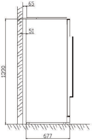
安裝側視圖
