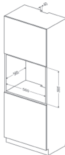
EB 13523 E 安裝尺寸圖
