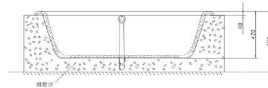
嵌入式安裝法
