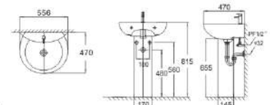
MAJI 麻吉 K-1137+K-1037 (不含龍頭)
