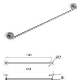
SB-1027 • 單桿毛巾架 (60公分) List Price: $ 2,000.
