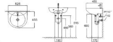
NIKE 尼克 K-1136+K-1037 (不含龍頭)
