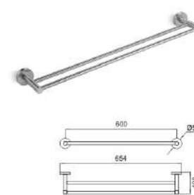
SB-1027D • 雙桿毛巾架 List Price: $ 2,800.
