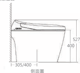
側面圖
