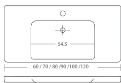
一體成型半嵌面盆(櫃體有假抽) -- 50831
