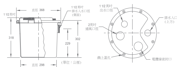
尺寸及安裝示意圖
