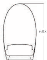
俯視圖
