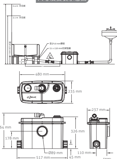
尺寸及安裝示意圖
