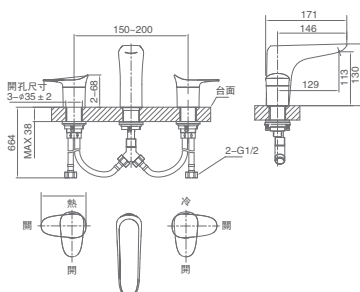
附：美規拉桿落水頭、高壓管、 三角凡爾、螺紋加長 P 管
