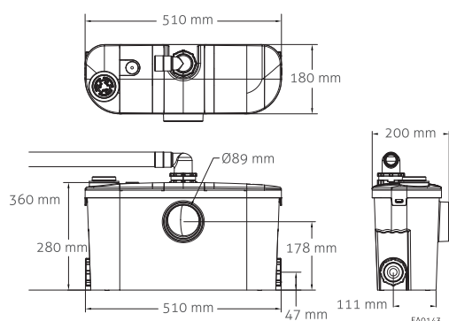
尺寸及安裝示意圖
