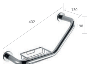
帶籃扶手 402x130x198mm
