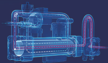
保溫層 第一層水路 第二層水路 環形加熱管
