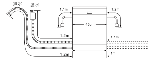
機體安裝尺寸:H820-880xW450xD580mm
