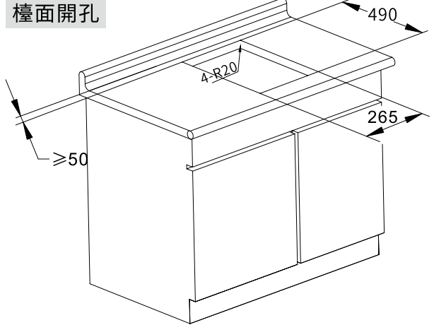
檯面開孔尺寸：265X490 4-R20
