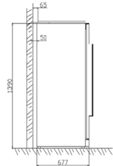
安裝側視圖
