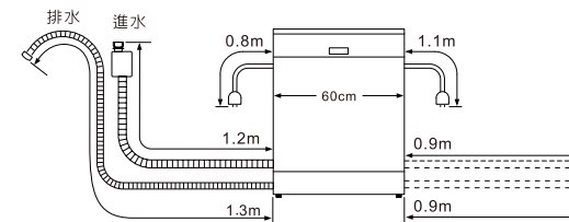
機體安裝尺寸:H820-880xW600xD580mm
