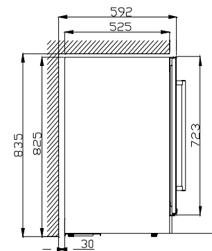
安裝側視圖
