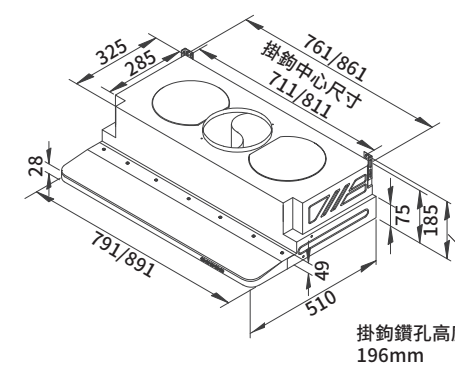
RH-8127/9127
