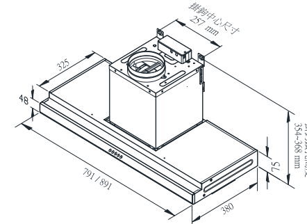
RH-8126E/9126E
