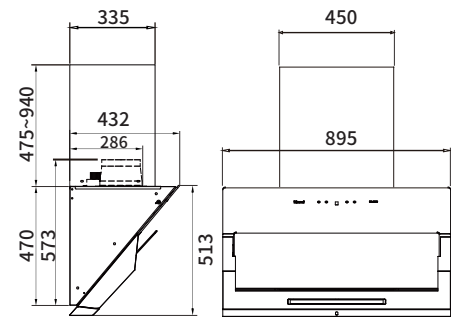
RH-9391R
