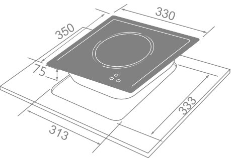
爐具底部與下方櫃體安裝空間需大於100mm(含)以上
