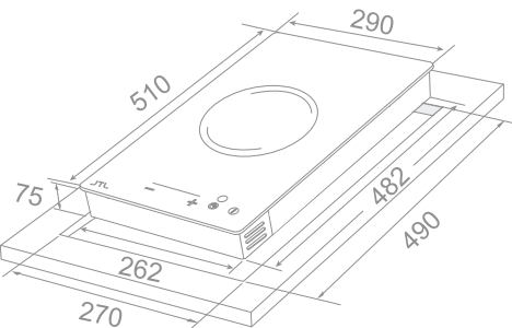
爐具底部與下方櫃體安裝空間需大於100mm(含)以上
