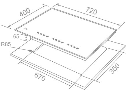
爐具底部與下方櫃體安裝空間需大於100mm(含)以上
