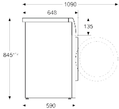
細部尺寸
