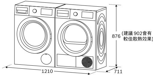
左右安裝
