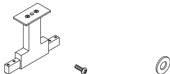
本体 F ×1 本体固定ネジ ×2 平座金 ×1
