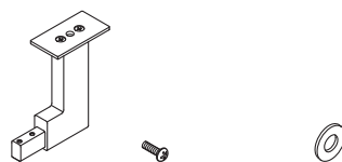
本体 E ×1 本体固定ネジ ×2 平座金 ×1
