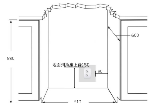
櫥下式紅酒櫃 預留空間尺寸圖
