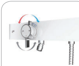
2 in 1 閥芯 TPS ( 預設溫度設計 ) 兩用閥芯。利用單一閥芯達到出水切換與分水器的功能，並可調整水溫。
