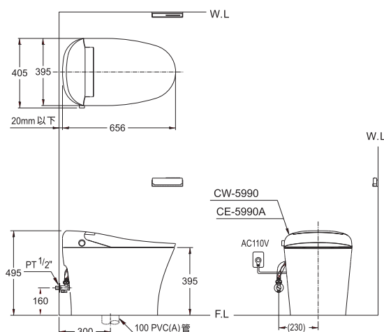
尺寸圖
