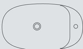
Art. 5408 SKINNY 70x40RL - 70x40 Cm - 16 Kg - 14 L.
