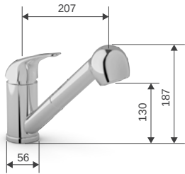
K1680001-TWQ 41 D259 x H187 Ø 56
