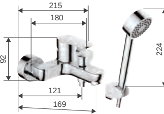
S5380101-TW Vogue 樂活 W215 x D188 x H107
