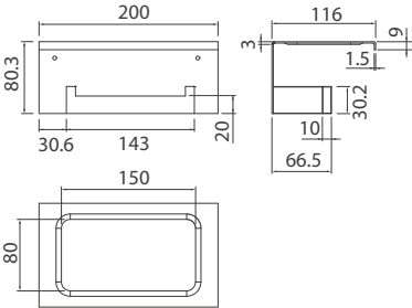
Y2382649-TW 43 Trim 魔方 帶置物功能紙巾架
