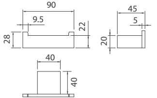
Y1782649-TW 43 Trim 魔方 掛衣鉤
