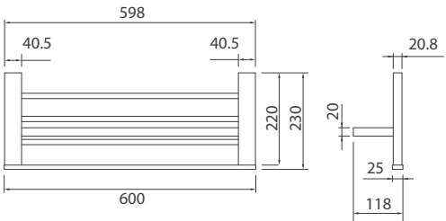
Y1382649-TW 43 Trim 魔方 帶置物功能毛巾桿
