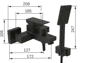
S5380549-TW Trim 魔方 消光黑 W208 x D185 x H101
