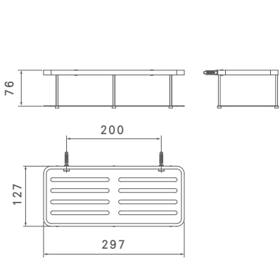
Y3380237-TW Y3380249-TW Rotunda 星動 不鏽鋼置物架
