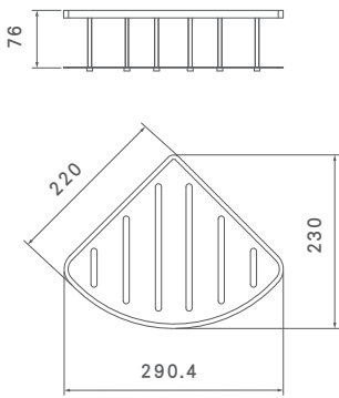
Y3280237-TW Y3280249-TW Rotunda 星動 不鏽鋼轉角藍
