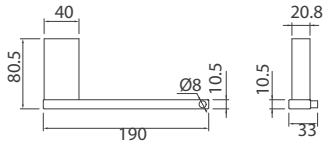
Y1482649-TW 43 Trim 魔方 毛巾桿
