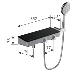
S5328901-TW 19 Jazz 爵士 單花灑 W350 x D156 x H100 牆面至浴缸出水口中心距離 D76
