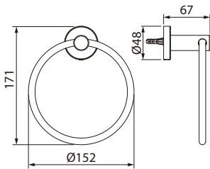
Y1480201-TW1 Y1480249-TW1 Rotunda 星動 毛巾環
