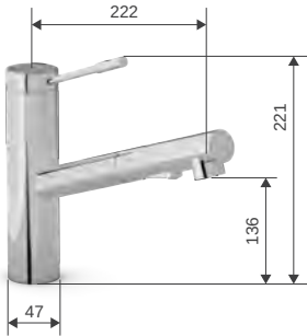
K1623901-TWPF1 41 D259 x H221 Ø 47
