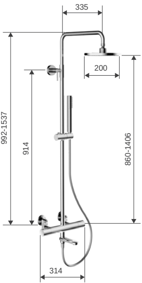
S5902401-TW 29 Splice 普萊斯 牆面至頂噴中心點距離 D437
