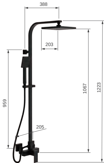
S5780549-TW Trim 魔方 消光黑 牆面至頂噴中心點距離 D388
