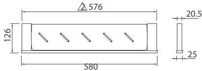
Y3182649-TW 43 Trim 魔方 置物架
