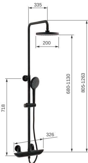
S5582449-TW Skitter 捷克 消光黑 牆面至頂噴中心點距離 D416.5
