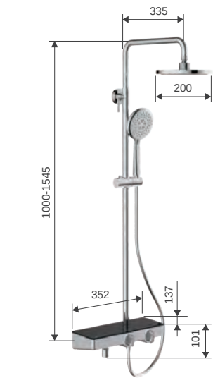
S5729001-TW 19 Jazz 爵士 雙花灑 牆面至頂噴中心點距離 D384 牆面至浴缸出水口中心距離 D76
