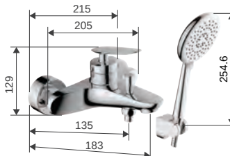
S5382401-TW Skitter 捷克 W215 x D206 x H130
