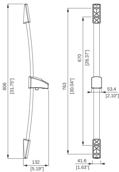
P1230101-TW1 P1230149-TW1 不鏽鋼升降桿
