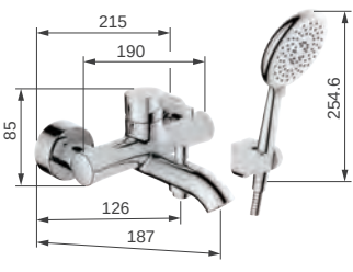
S5381601-TW Glide 加德 W215 x D198 x H109
