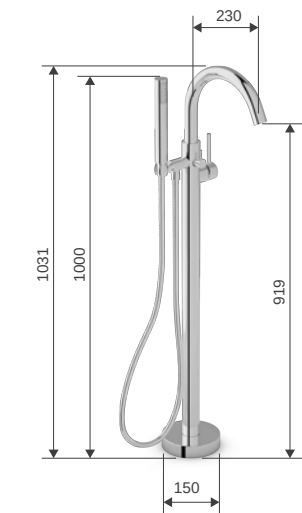
S7660701-TW 35 Rotunda 星動 本體中心點至出水口中心點距離 D230
