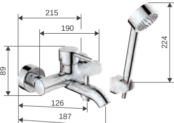
S5381201-TW1 Glide 加德 W215 x D198 x H113
