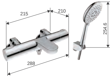
S5402401-TW1 Splice 普萊斯 W288 x D210 x H100 牆面至浴缸出水口中心距離 D191
