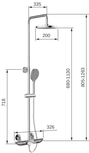
S5882401-TW 24 Skitter 捷克 牆面至頂噴中心點距離 D416.5
