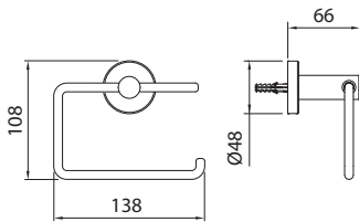
Y2380201-TW2 Y2380249-TW2 Rotunda 星動 紙巾架
