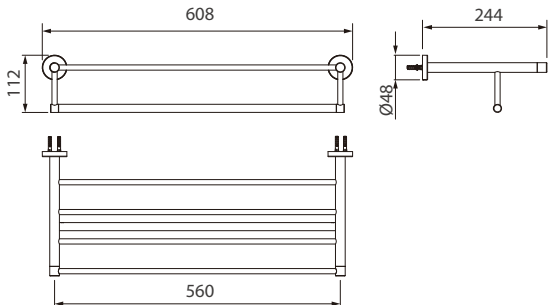
Y1380201-TW1 Y1380249-TW1 Rotunda 星動 雙層毛巾桿
