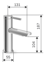
W8129101-TW4 33 Glide 加德 D178 x H187 Ø55
