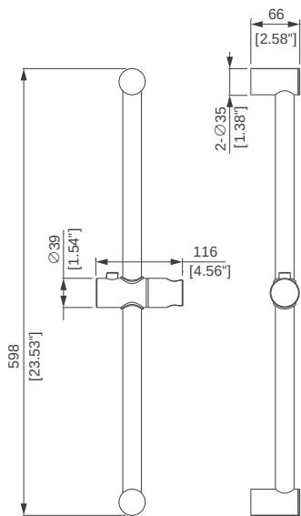
P0230401-TW1 P0230449-TW1 不鏽鋼升降桿
