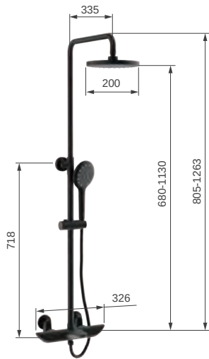
S5882449-TW 24 Skitter 捷克 消光黑 牆面至頂噴中心點距離 D416.5
