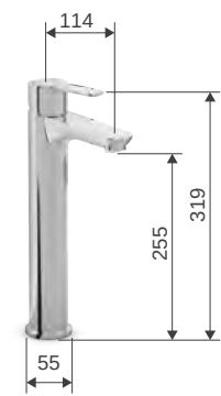
W3581301-TW4 27 Splice 普萊斯 D157 x H319 Ø55
