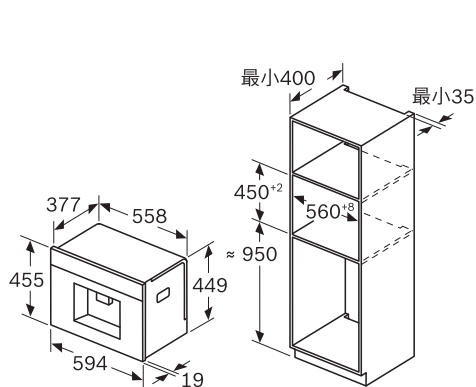
櫃體400mm深
