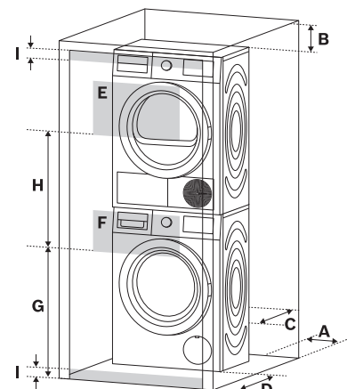
櫥櫃內堆疊安裝
