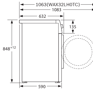
細部尺寸
