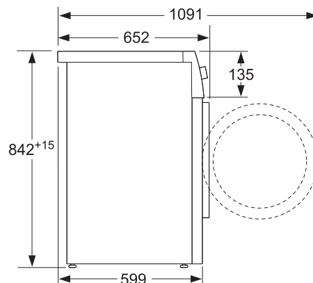
左右安裝
