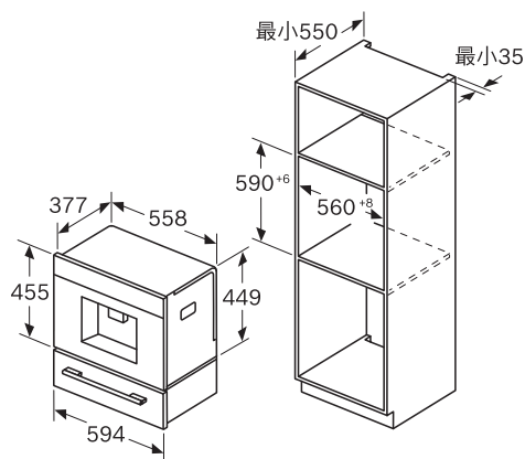
櫃體550mm深
