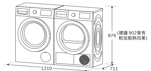
左右安裝
