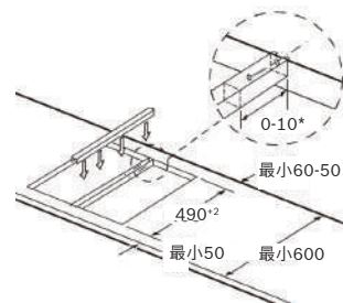
連接條安裝圖
