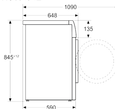
細部尺寸
