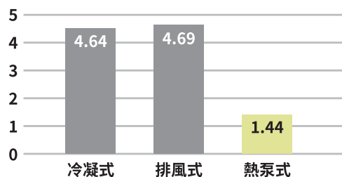
各式烘衣機耗電量比較表 (Kwh/cycle)
