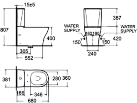
Cygnet 分體馬桶 CL26255-6DACTCB 定價 $34,000
