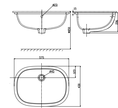
Activa 下嵌型面盆 580mm CCAS0426-1000410F0 定價 $4,300
