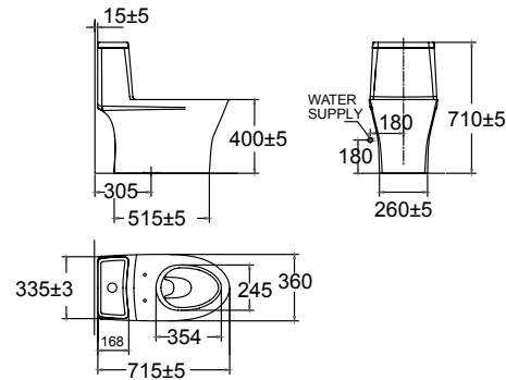
Flexio 單體馬桶 CL25300-6DACTST 定價 $31,200
