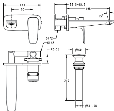
Signature 壁出面盆龍頭 FFAS1704-1015LOBCO 定價 $18,400
