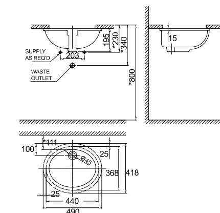
Ovalyn 下嵌型面盆 490mm CCAS0470-1000410F0 定價 $4,300
