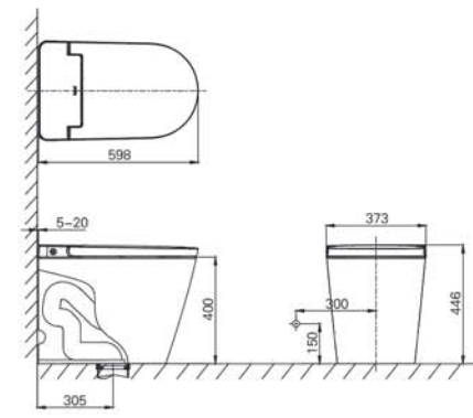
ENC2179UW-3 一體座便器 尺寸: 598x373x446mm 蓋板: UF緩降薄蓋板 坑距:305mm 名義用水量: 4.2/6L 沖水系統:虹吸
