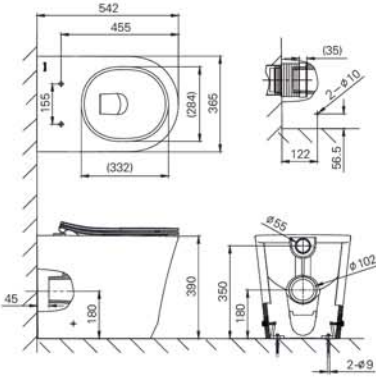
ENC2175UW 落地式座便器 尺寸: 542x365x390mm 蓋板: UF緩降薄蓋板 坑距: H=180mm (P排) 可搭配NCD03C隱藏式水箱使用 沖水系統:直沖
