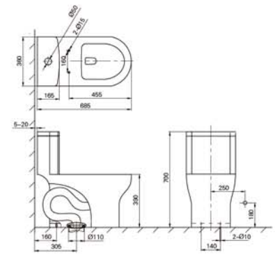
ENC2155JW-3 連體座便器 尺寸: 685x360x700mm 蓋板: PP緩降蓋板 坑距: 305mm 名義用水量: 3/4.5L 沖水系統:虹吸
