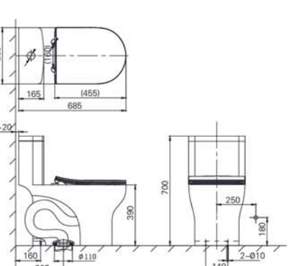
ENC2155JW-3T0 連體座便器 尺寸: 685x360x700mm 蓋板: PP緩降蓋板 坑距: 305mm 名義用水量: 3/4.5L 沖水系統:虹吸
