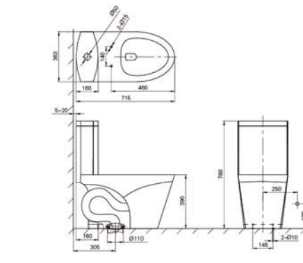
ENC2156JW-3 連體座便器 尺寸: 715x363x780mm 蓋板: PP緩降蓋板 坑距: 305mm 名義用水量: 3/4.5L 沖水系統:虹吸
