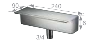
A-207-6 浴缸瀑布出水 ( 隱藏式 ) Concealed Waterfall Spout
