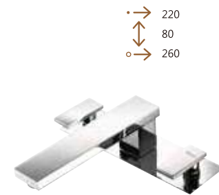
A-8562-3 (三件式) 浴缸龍頭 3- Hole Tub Faucet
