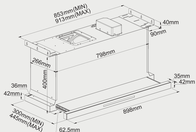
機型 423L
