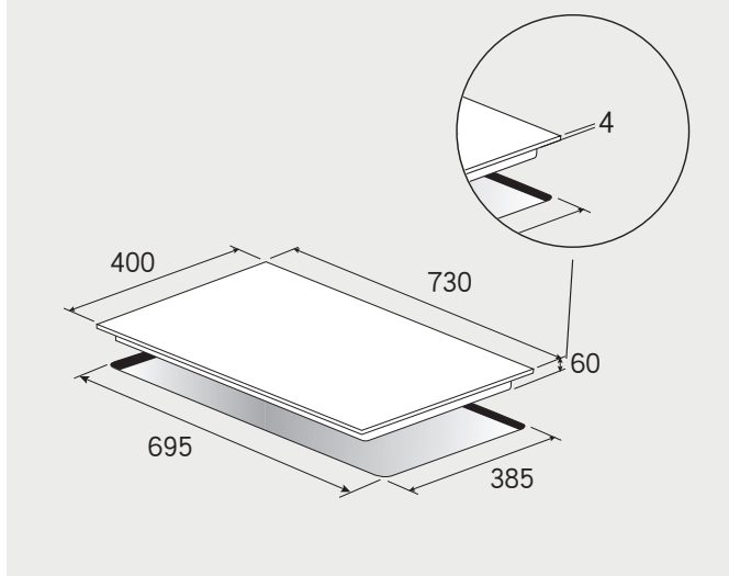
感應爐安裝散熱圖
