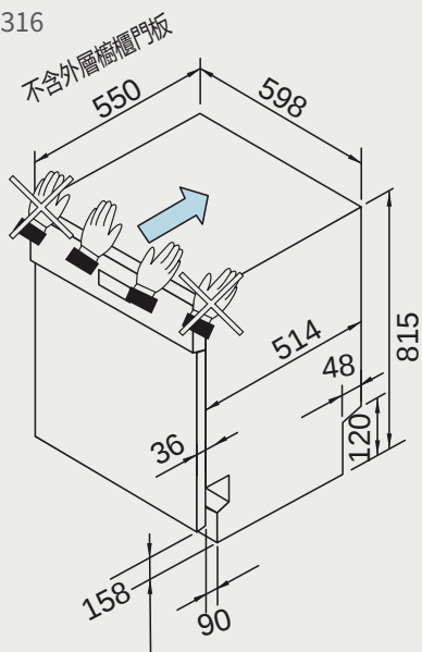
機型 G2316
