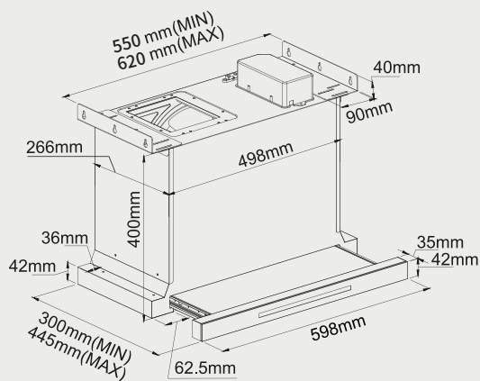
機型 423
