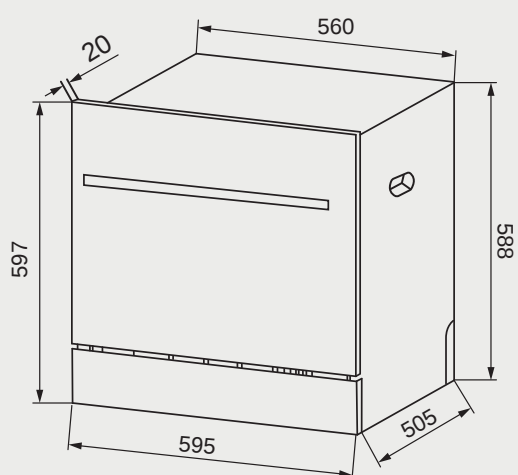
機型 G2510
