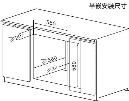
半嵌安裝尺寸
