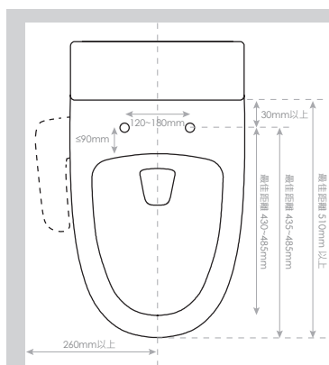
HE-0625 / HE-0525 安裝建議
