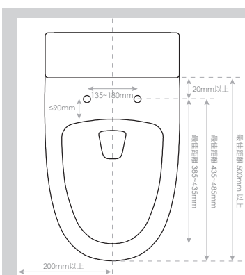
HE-0515 安裝建議
