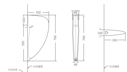
U-2800 小便斗隔板 NT 4,600 尺寸 350x100x760mm
