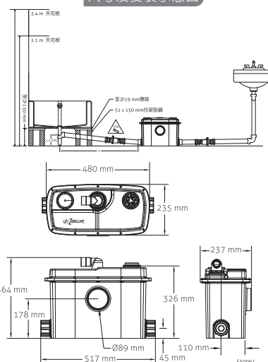
尺寸及安裝示意圖
