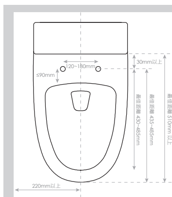
HE-0635 / HE-0535 安裝建議
