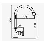
D-1206 MBR 工業風長栓附起泡器 Single Cold Tap 2025-1670
