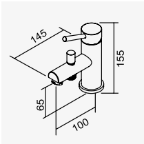
D-90287 鉻色 沐浴/面盆兩用龍頭 Shower & Basin Faucet D-564 陶瓷心軸 35L 低腳 搭配單段式蓮蓬頭 全套零件附按壓式落水頭 2025-7670
