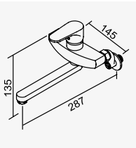
D-9028 鉻色 廚房/浴缸龍頭(出水管20cm) Kitchen/Bath Faucet D-563 陶瓷心軸 35H 高腳 2025-6170
