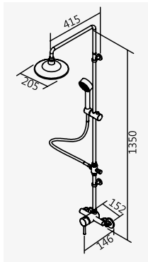
D-5166 鉻色 SPA沐浴龍頭 Rain Shower Faucet D-562 陶瓷心軸 40L 低腳 3-5公斤水壓 搭配單段式蓮蓬頭 2025-8340
