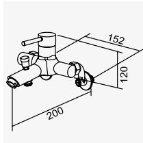
D-80255 鉻色 沐浴龍頭 Shower Faucet D-563 陶瓷心軸 35H 高腳 搭配單段式蓮蓬頭 2025-6000
