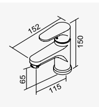
D-9088 鉻色 面盆龍頭 Basin Faucet D-840 西班牙SEDAL閥芯 35 高腳 全套零件附按壓式落水頭 2025-6170
