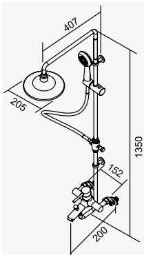
D-9355 鉻色 SPA沐浴龍頭 Rain Shower Faucet D-563 陶瓷心軸 35H 高腳 3-5公斤水壓 搭配單段式蓮蓬頭 2025-13340
