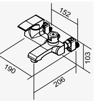
D-9167 鉻色 沐浴龍頭 Shower Faucet D-563 陶瓷心軸 35H 高腳 搭配三段式蓮蓬頭 2025-9340
