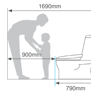
傳統低水箱式馬桶
