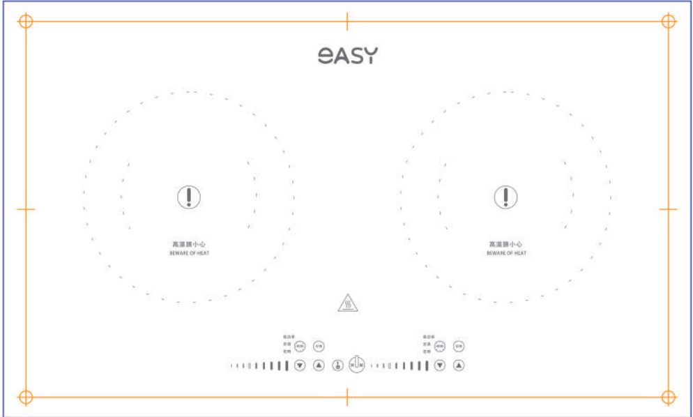
上嵌式挖孔圖 (設備面板高於桌面) 挖孔尺寸： 寬680 x 深400 x 高109 mm
