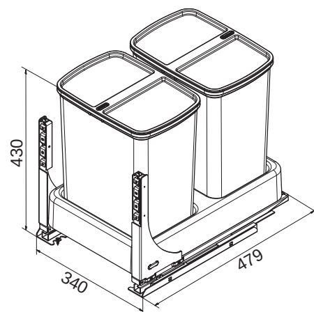
示意圖 / 門板孔位圖 Schematic / Door Hole Location Diagram
