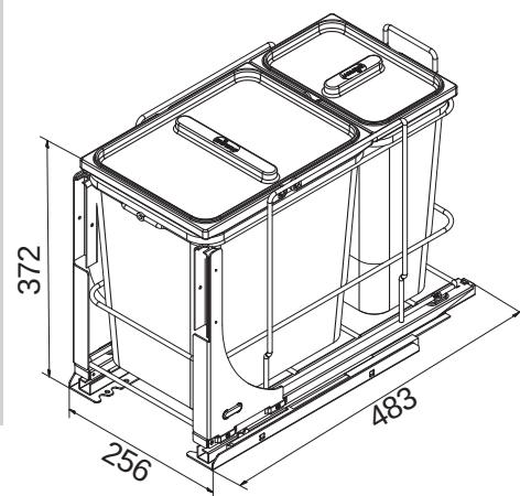
示意圖 / 門板孔位圖 Schematic / Door Hole Location Diagram
