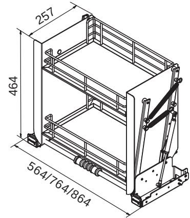
示意圖 Schematic
