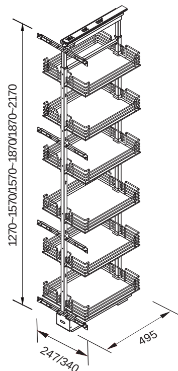
示意圖 Schematic
