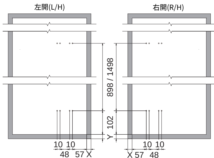
門板孔位示意圖
