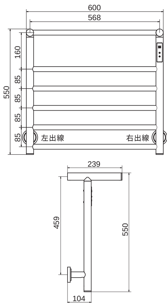
示意圖 Schematic
