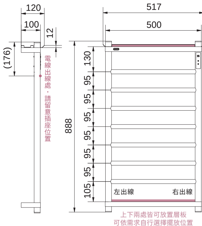
示意圖 Schematic
