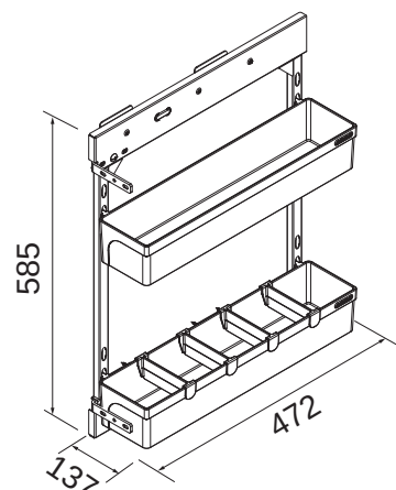
示意圖 Schematic
