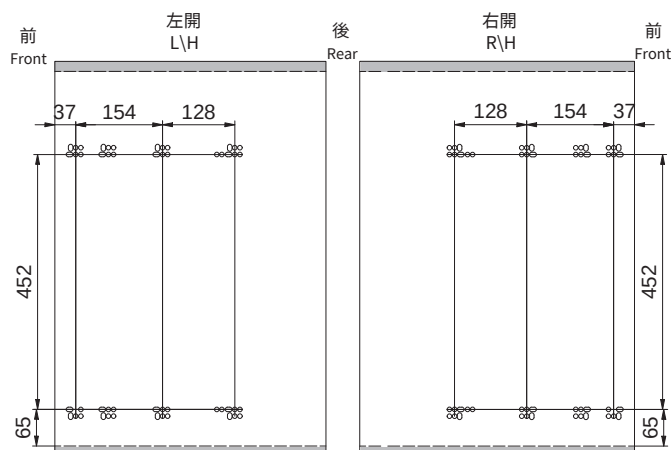
側板孔位圖 Sidewall Schematic
