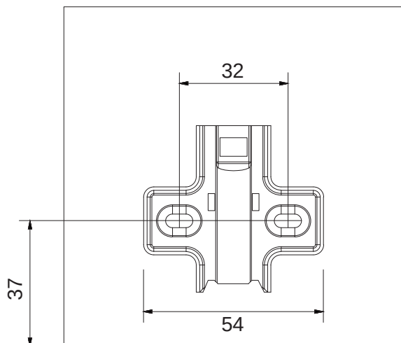
二孔底座 Hinge Mounting Plate, 2 Holes
