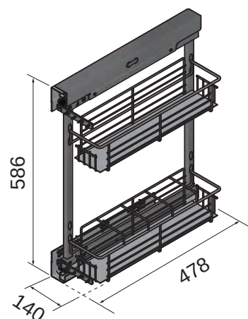
示意圖 Schematic
