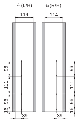
底板尺寸圖
