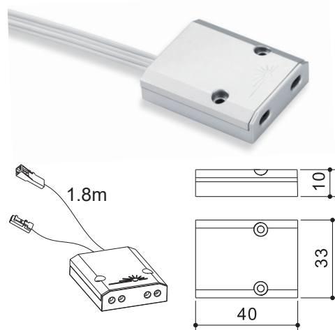
雙紅外線感應開關 Dual IR Sensor Switch
