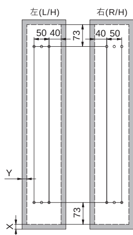
門板尺寸圖
