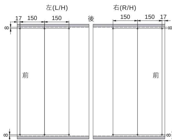
側板尺寸圖
