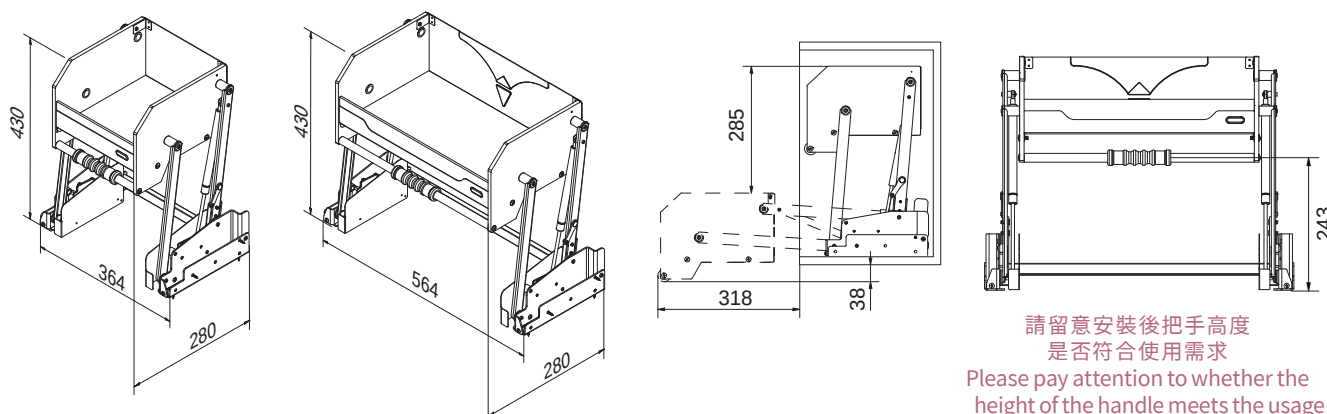
示意圖 Schematic
