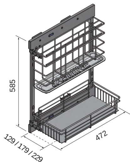
示意圖 Schematic
