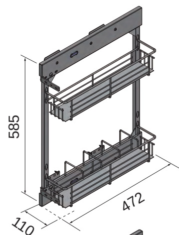
示意圖 Schematic
