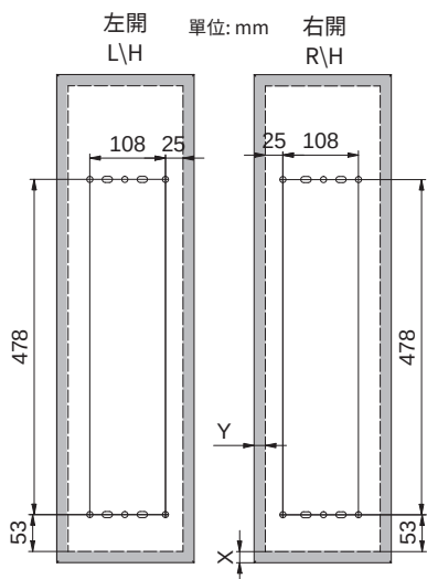
門板孔位圖 Door Panel Schematic
