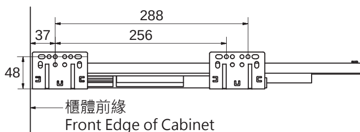
滑軌孔位圖
