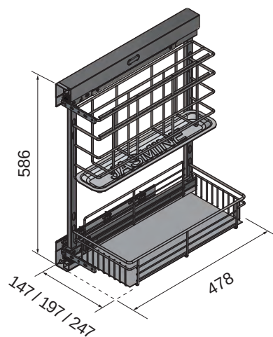
示意圖 Schematic
