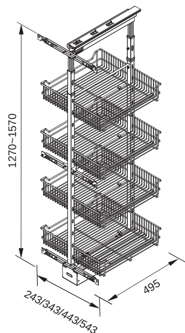
示意圖 Schematic
