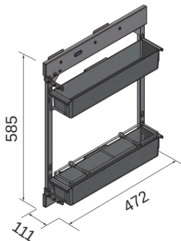
示意圖 Schematic
