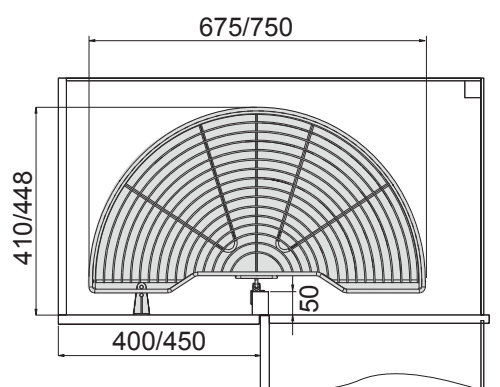
示意圖 Schematic
