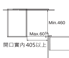
開啟角度與相鄰櫃體示意圖
