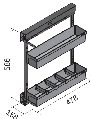
示意圖 Schematic
