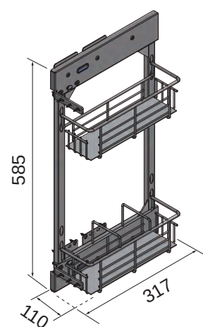
示意圖 Schematic
