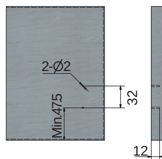
門板孔位 Holes of Drilling Dimension
