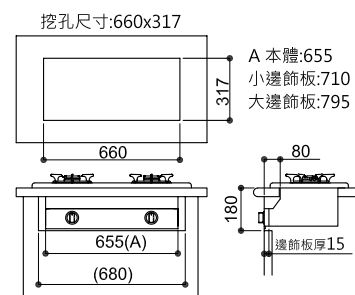
RBTS-L260S 嵌入式彩焱不鏽鋼雙口爐
