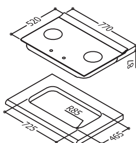
RB-L2710G(B) 檯面式彩焱玻璃雙口爐
