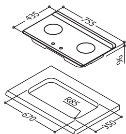
RB-L2600S 檯面式彩焱不鏽鋼雙口爐
