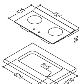
RB-L2680G(B) 檯面式彩焱玻璃雙口爐
