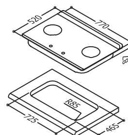
RBTS-L260S 嵌入式彩焱不鏽鋼雙口爐
