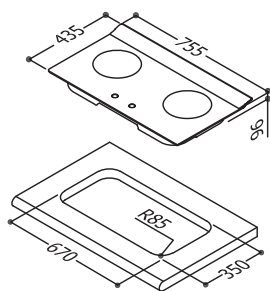
RB-L2620G(B) 檯面式彩焱玻璃雙口爐
