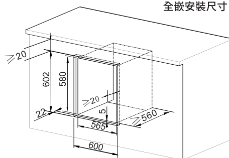
全嵌安裝尺寸
