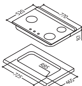
RTS-L270S 台爐式彩焱不鏽鋼雙口爐
