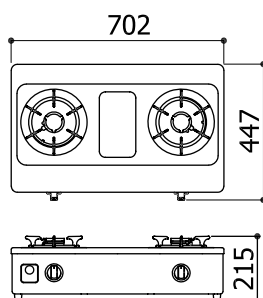
RTS-L270S 台爐式彩焱不鏽鋼雙口爐
