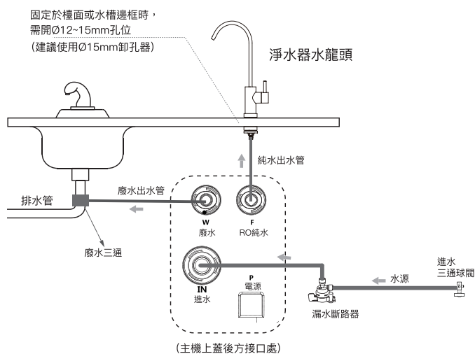
純水RO安裝尺寸圖
