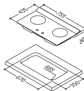
RB-L2600G(B) 檯面式彩焱玻璃雙口爐
