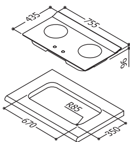
RB-L2610G(B) 檯面式彩焱玻璃雙口爐
