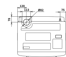
RDT-90-TR-W
