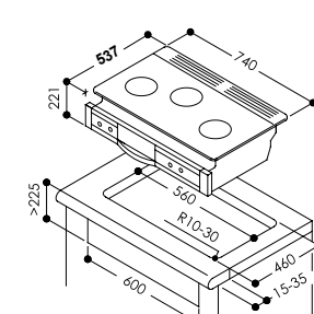
RBG-N71W5GA3X-SVL-TR
