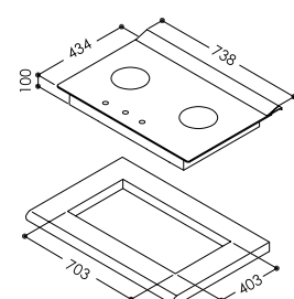
RB-2CGT-TR
