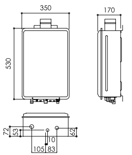
REU-A2426WF-TR
