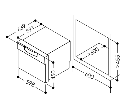
RKW-601C-SV-TR
