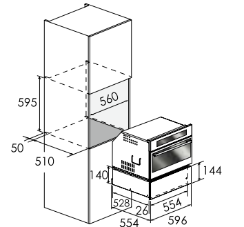
RKW-601C-SV-TR
