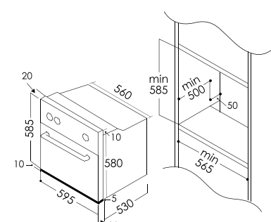
RBO-5CS1-TW
