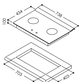
RB-2CGN-TR
