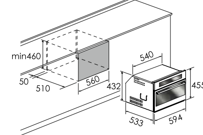
RBSO-970
