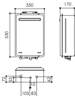
REU-A2426W-TR
