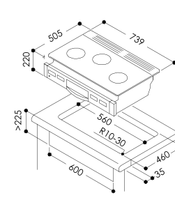
RB71AM5U32S-VW-TR RB71AM5U32R-VW-TR
