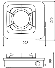
RTS-1ND
